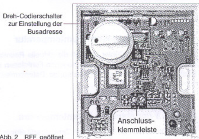
Abb. 2 RFF geöffnet
